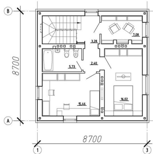
План 2-ого поверху
